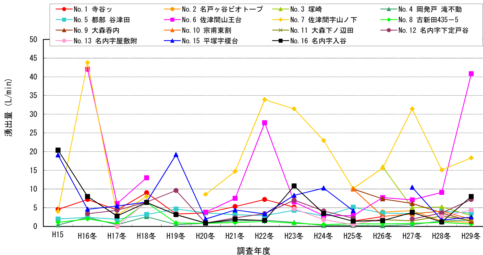
図 2-3 地点別湧出量の推移（冬季）
