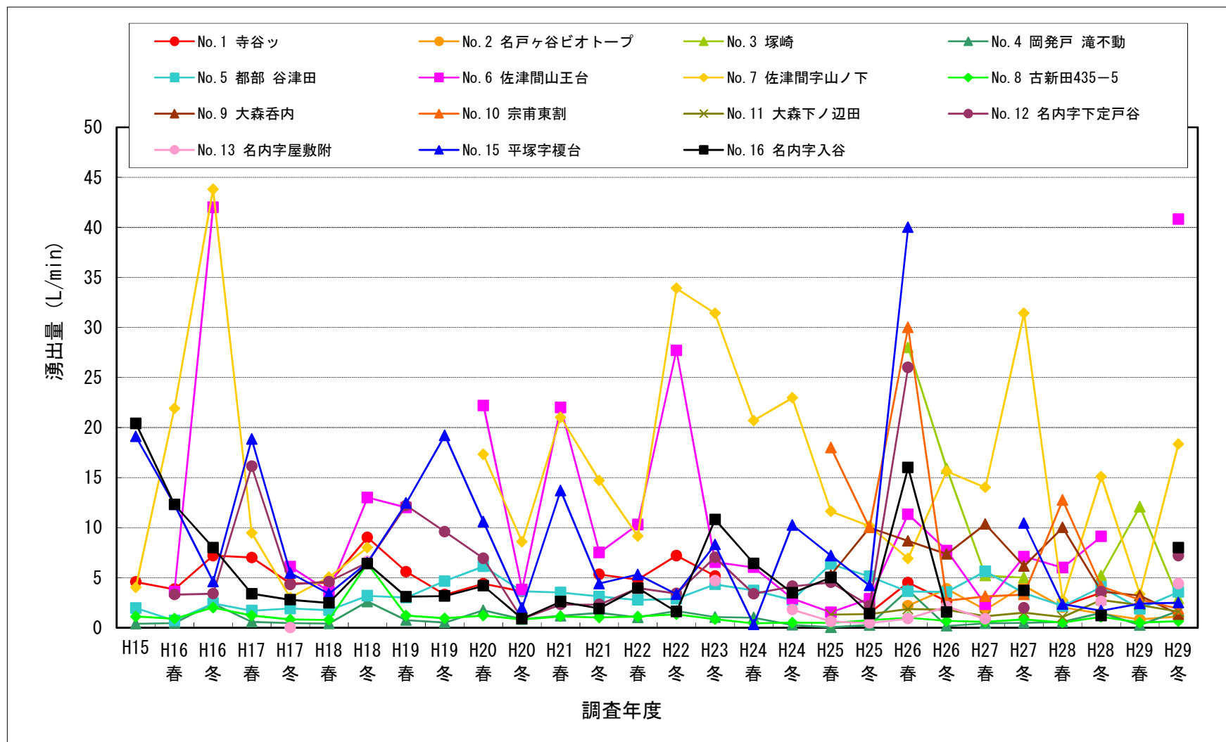
図 2-1 地点別湧出量の推移 注) H17 年度春の No. 6、H19 年度春の No. 7、H22 年度春・冬の No. 13 は湧出量が多すぎて測定不能。H26 年度春・冬の No. 4 は測定地点での湧出量が 0 であったため、測定地点を変更。H27 年度春の No. 1 は斜面下の広い範囲、No. 12、15、16 は水面下で湧出しているため測定不能。H27 年度冬の No. 1 は斜面下の広い範囲から、No. 13 は複数の場所からの湧出により測定不能。No. 14 は H27 年度から湧水が確認できず測定地点より除外。H28 年度春の No. 3 は湧出量が少なく、No. 12、No. 16 は複数の場所から湧出、No. 13 は湧出点不明のため測定不能。H29 年度春の No. 1、No. 6 は湧水量不足、No. 12、No. 16 は複数の場所から湧出、No. 13 は湧出点が不明のため、測定不能。H29 年度冬の No. 1 は湧水量不足のため測定不能。
