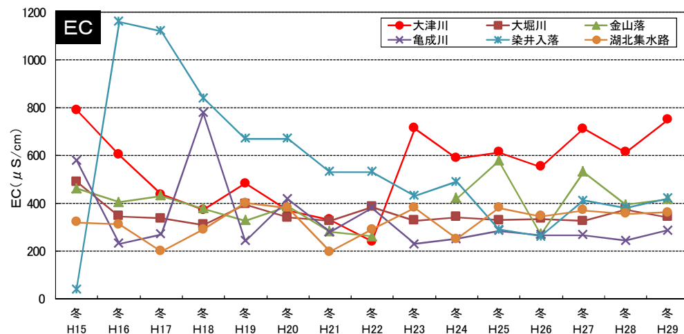
図 2-8 河川別年平均値の推移 (EC)
