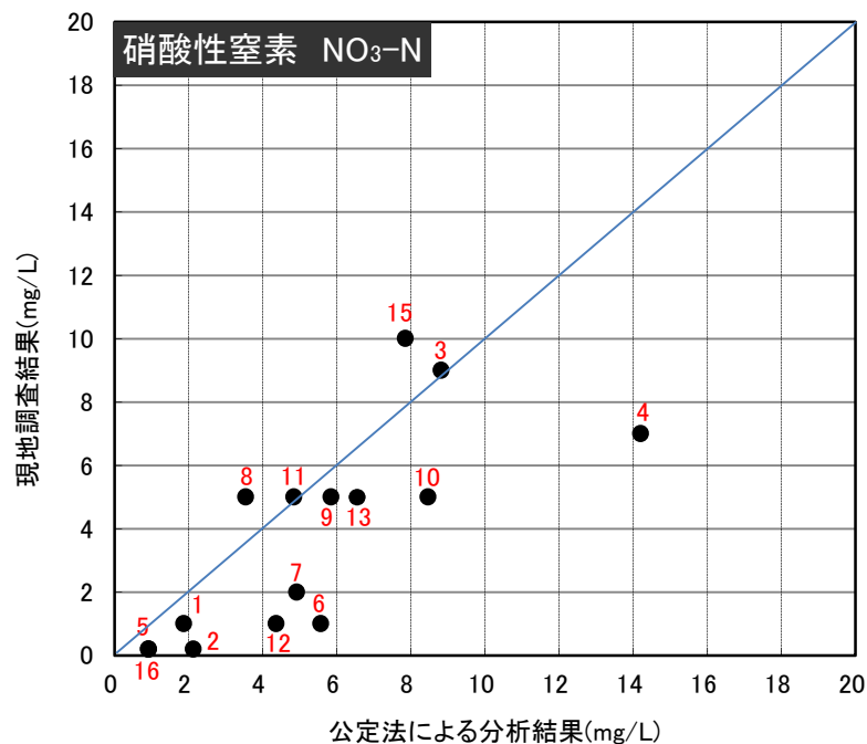
図 2-5 公定法による分析結果と現地調査結果の比較（冬季：硝酸性窒素）
