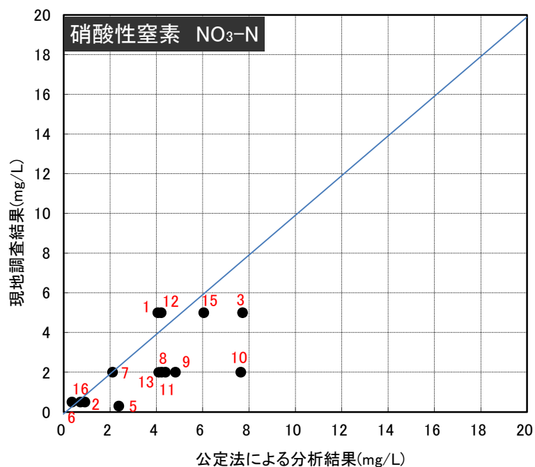
図 2-4 公定法による分析結果と現地調査結果の比較（春季：硝酸性窒素）
